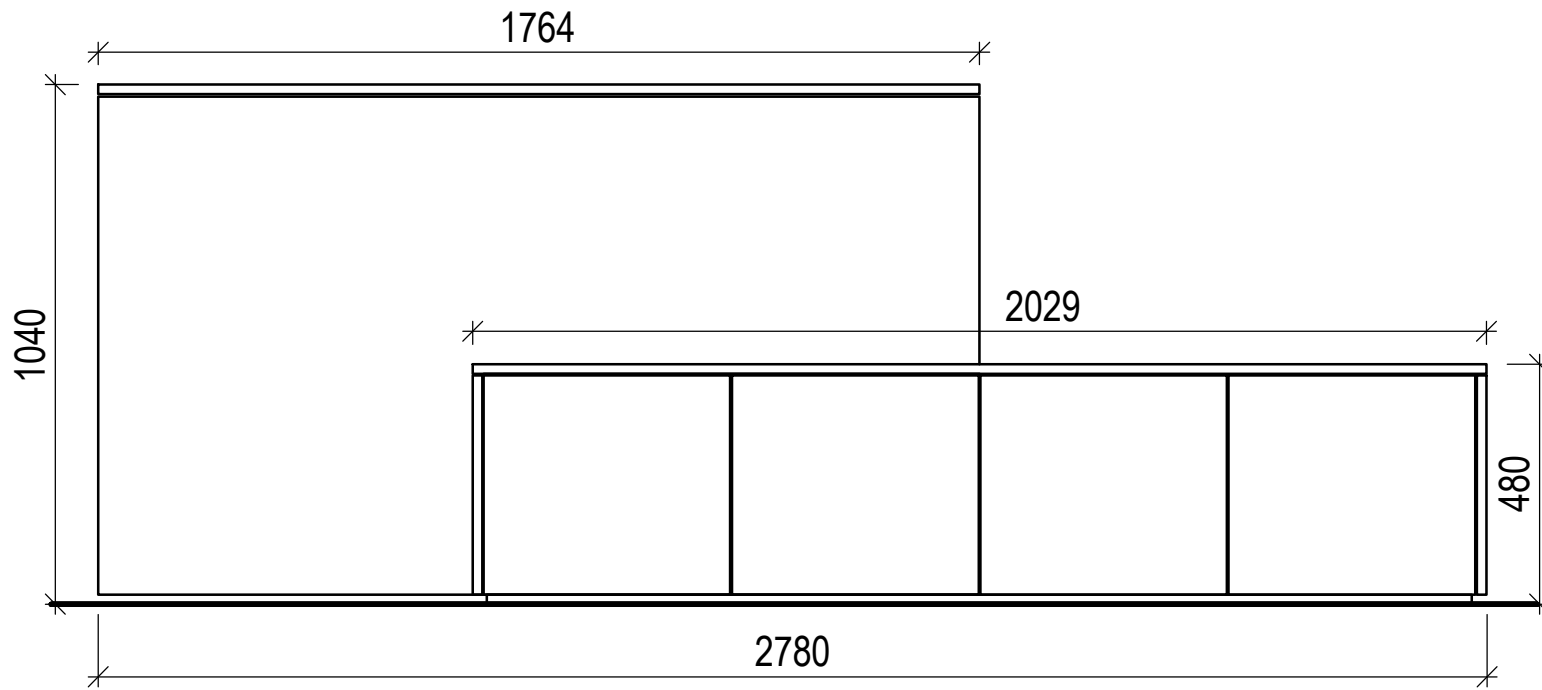
Ansicht Front
